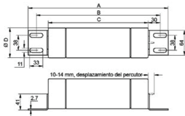
Placas de contacto tipo "F"
