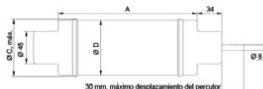
Fusibles EJ
