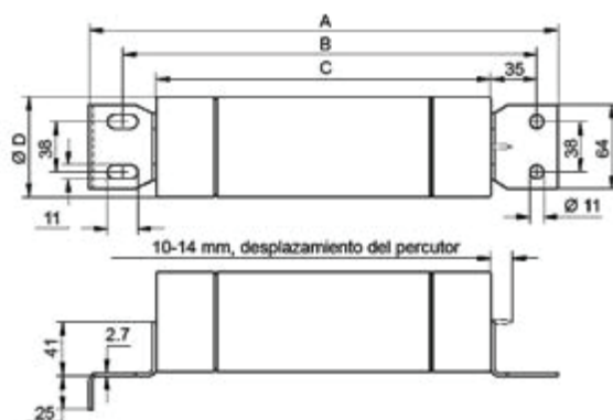
Placas de contacto tipos "C" y "D"
