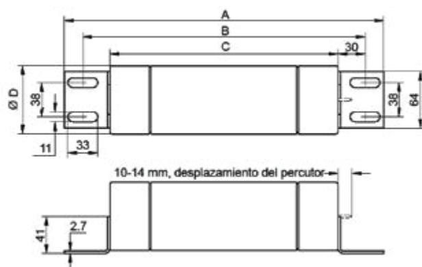
Placas de contacto tipo "F"
