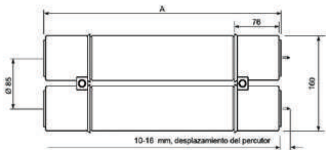
Placa de contacto tipo "K" (fusibles de doble barril)
