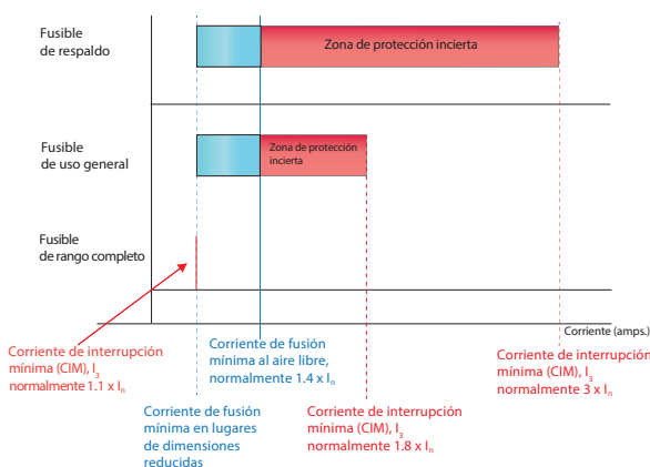
Funcionamiento de los fusibles de media tensión según la Norma IEC 60282-1
