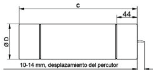
Placas de contacto tipo "A" (casquillo)
