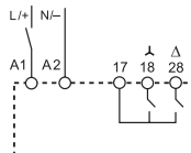
Esquema de conexión (sin señal de mando)
