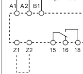
Esquema de conexión (con señal de mando)
